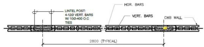
S1 LINTEL POST DETAIL 03 SCALE: N.T.S.
