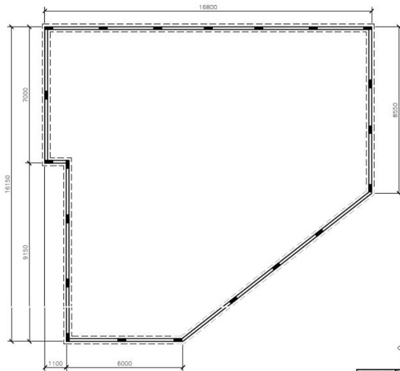
S1 BUNDWALL LAYOUT PLAN 01 SCALE: 1:200 mm
